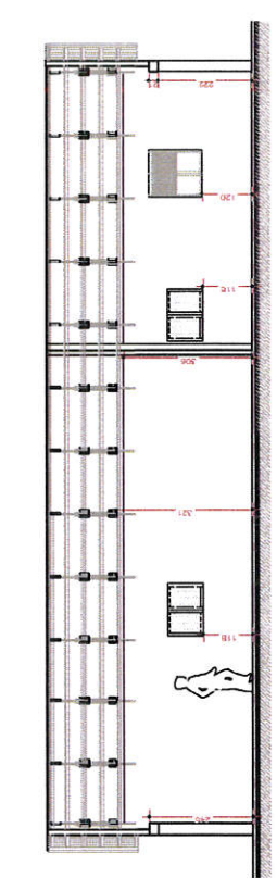
SEZIONE TRASVERSALE
